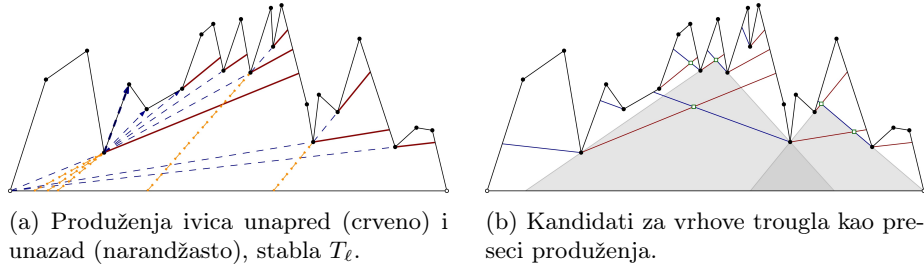
Slika 2: Produženja ivica i skup kandidata za vrhove utemeljenog trougla (preuzeto iz [1]).
